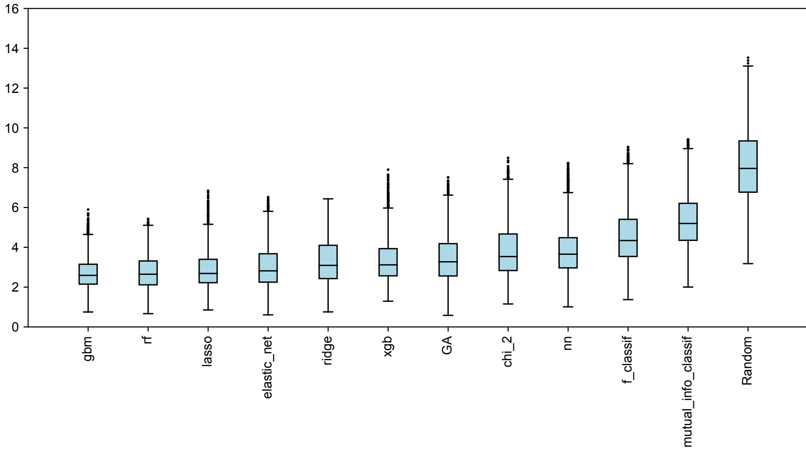
Mean NMF KL divergence
